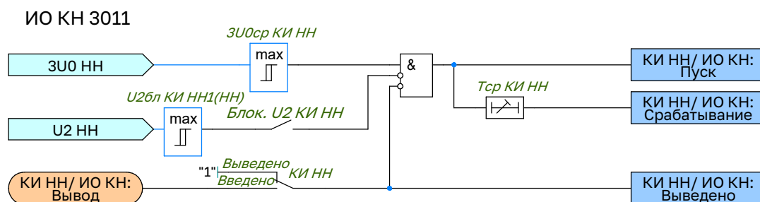
Рисунок 2.22 – Функциональная схема логики КИ НН
