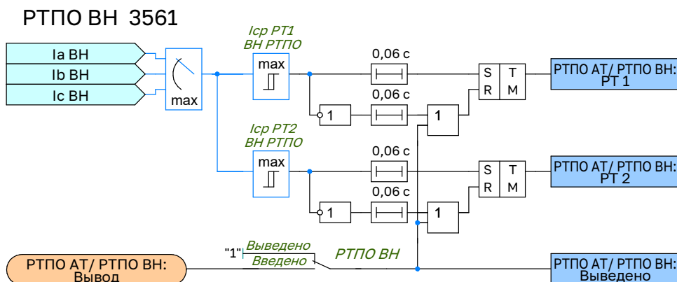
Рисунок 2.18 – Функциональная схема логики РТПО ВН
