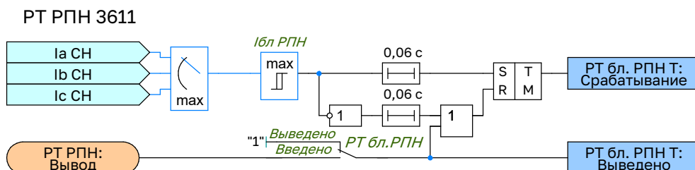
Рисунок 2.19 – Функциональная схема логики токового органа блокировки РПН
