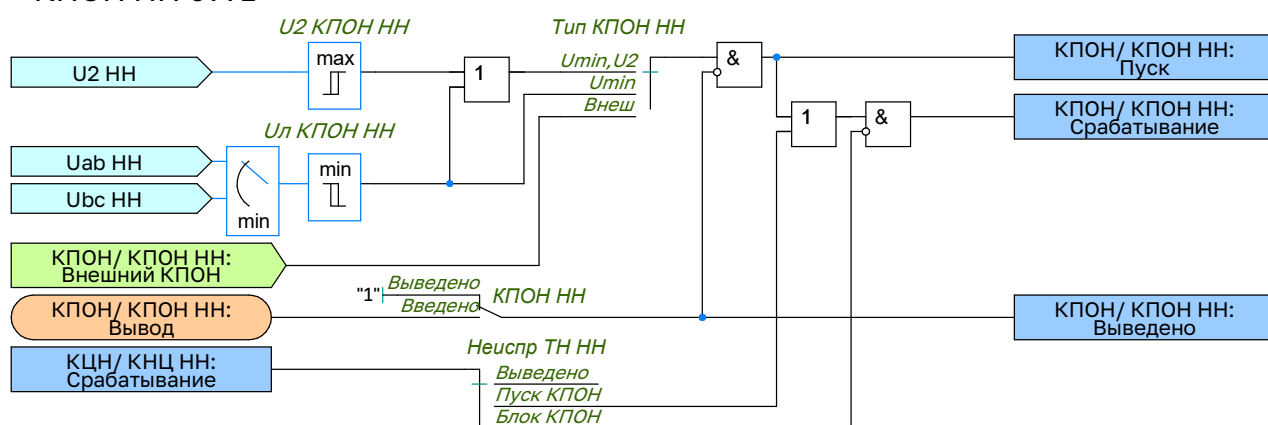
Рисунок 2.10 – Функциональная схема логики КПОН
